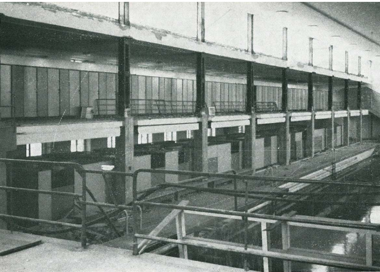
Blick auf die Nordseite der Wellenbadhalle, aufgenommen von der Gymnastik- und Sprungpore aus. Wir erkennen die vom Mauerwerk befreiten Träger.
