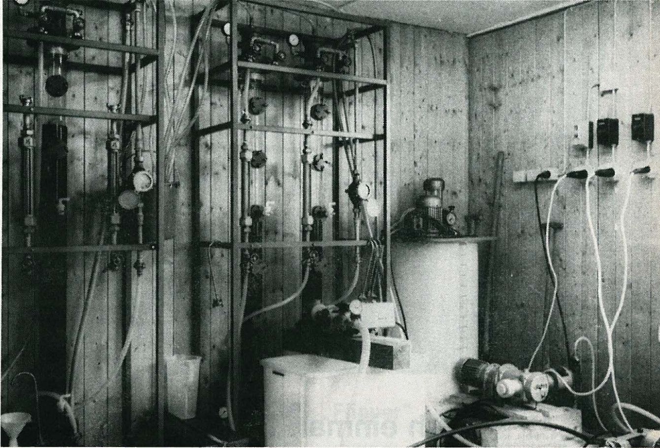
Teilblick in den Filterraum der Forschungsanlage mit seinem Gewirr von Leitungen und vielen Pumpen
